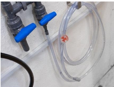
Tappeudstyr med to afgange. På den ene er monteret slange med automatisk stopfunktion, som sikrer den rette mængde vand til batteriet.
